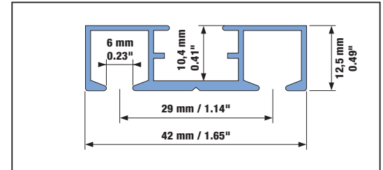
2 Maßstab / Echelle / Scale 1:1
