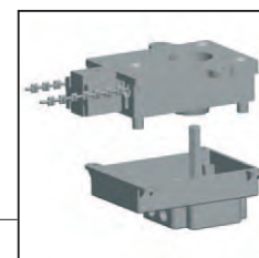
3135 932- Getriebeset / Tête entraînement / Head Pulley
