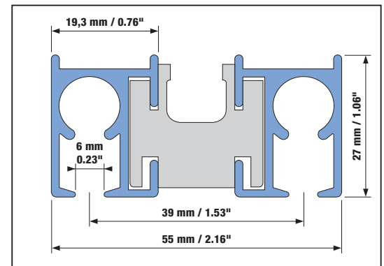
4 Maßstab / Echelle / Scale 1:1
