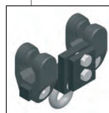
3105 0011 Zugwagen / Chariot conducteur / Master Runner
