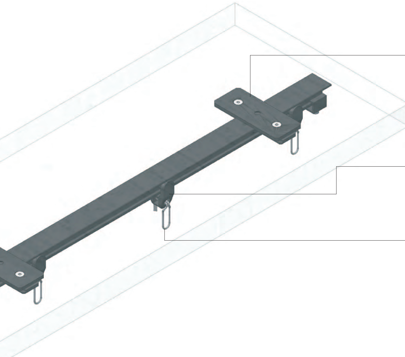
3100 8021 Deckenmontageplatte, schwarz / Fixation plafond, noir / Ceiling Mounting Plate, black
