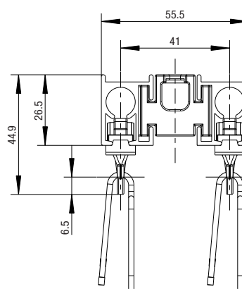
Seilzugschiene / Entraînement manuel par drisse / Internal rope drawn track
