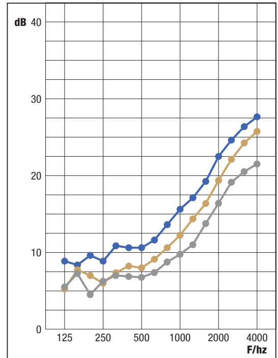
Schalldämm-Maße / Indices d'affaiblissement acoustique / Sound reduction factor
