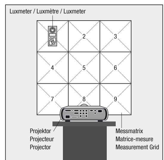
Messung des ANSI-Lumen / Mesure des ANSI-Lumen / ANSI-Lumen Test
