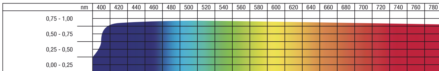
Farbspektrum Reflektionsgrad / Spectre lumineux Degré de réflexion / Colour Spectrum Degree of Reflection
